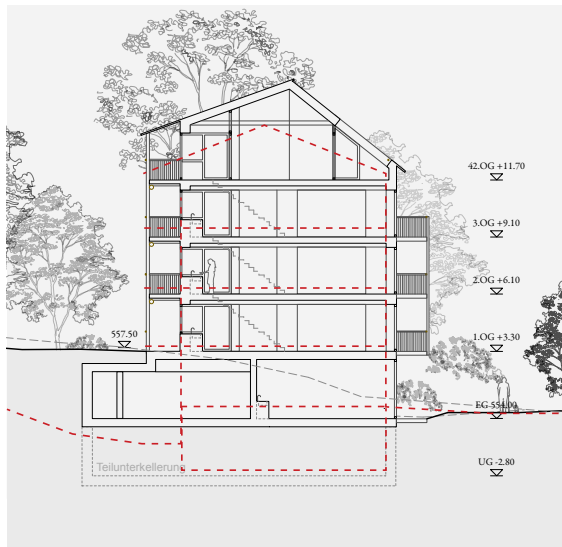
Schnitt E (aktueller Stand)
