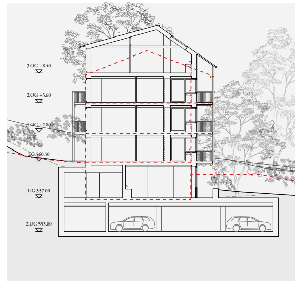
Schnitt D (aktueller Stand)
