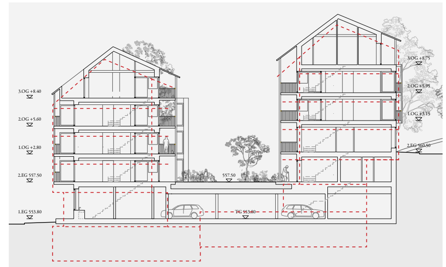
Schnitt B/C (aktueller Stand)
